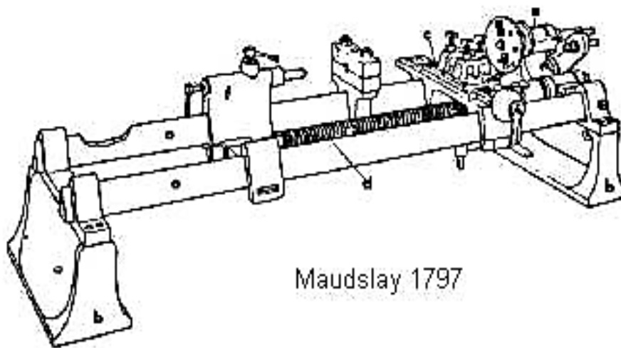
Рис. 2. Станок с крестовым суппортом Генри Модсли
