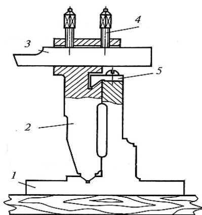
Рис. 1. Схема суппорта Нартова (1714)
