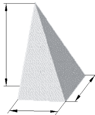
ПИРАМИДА
