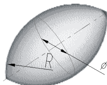
САМОПЕРЕСЕКАЮЩИЙСЯ ТОР
