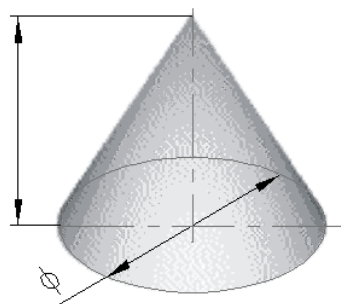
КОНУС
