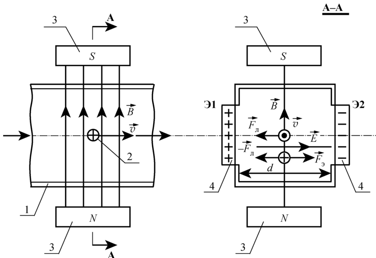
Рис. 4. Принципиальная схема индукционного датчика расхода: 1 – канал с протекающей жидкостью; 2 – заряженная частица жидкости; 3 – полюсные обкладки электромагнита; 4 – электроды (Э1 и Э2)
